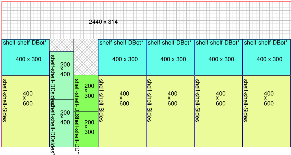
Layout 3 of 9(Stock:stk1 Dim:2440 x 1220 Qty:1 Material:mdf Thk:10)
